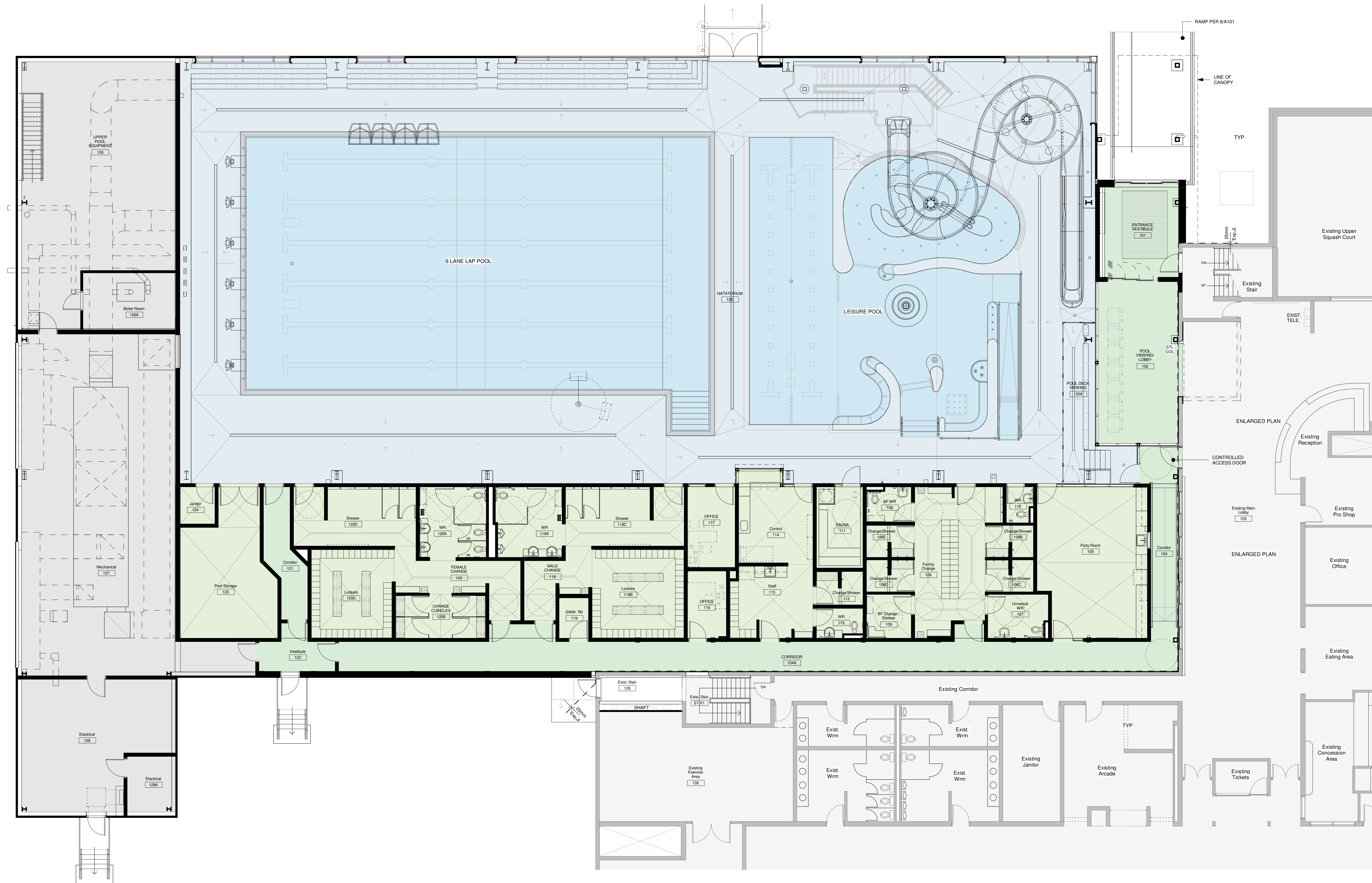
1 Level 1 - Natatorium P2 1 : 100
